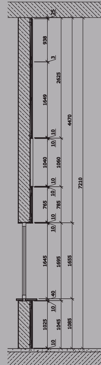
Schnitt F-F M 1/20
